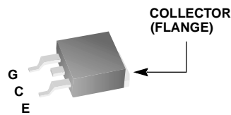
JEDEC TO-263AB
